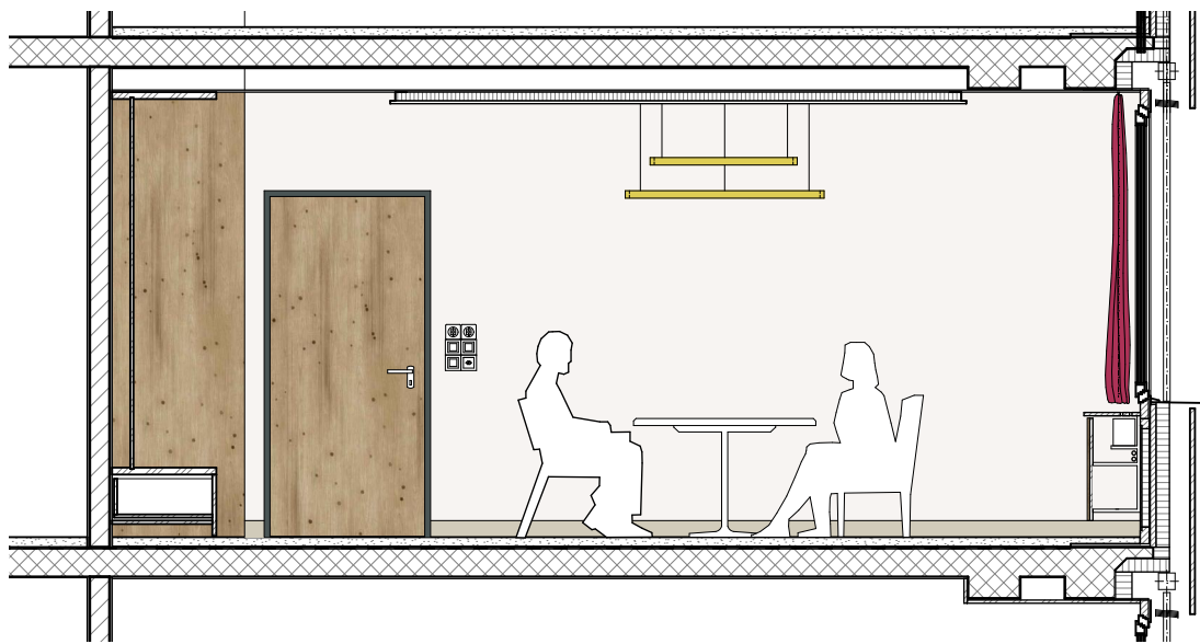
INNENANSICHT WEST
