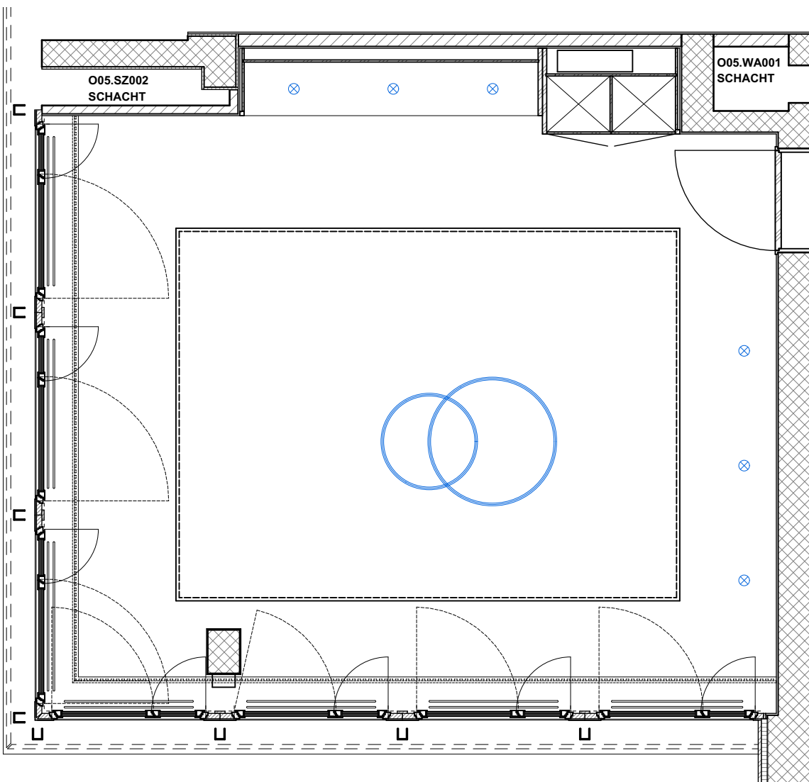
DECKENSPIEGEL
