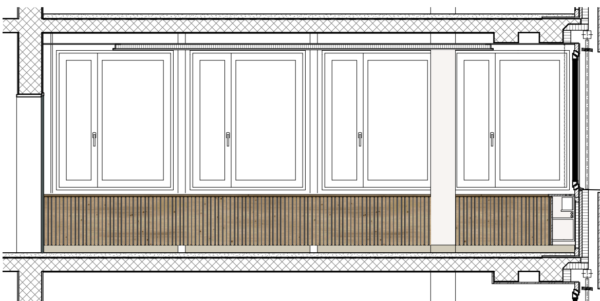
INNENANSICHT NORD
