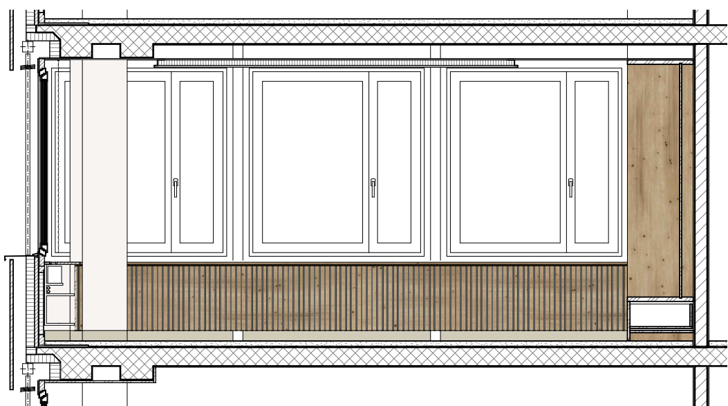
INNENANSICHT OST
